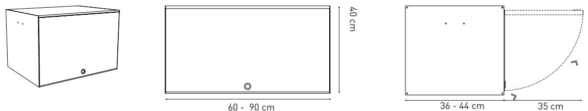
Ribaltina, apertura dal basso / Hanged tip-up panel, opening from the bottom
